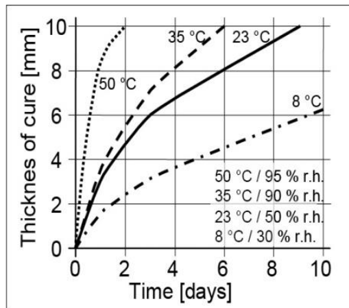
1 grafikas. SikaTack® Panel-50 stingimo greitis
